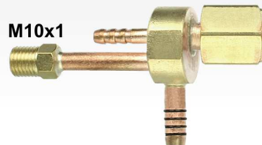
ESAB - ZA Strom/Wasserweiche
