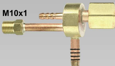
ESAB - ZA mit Strom/Wasserweiche
