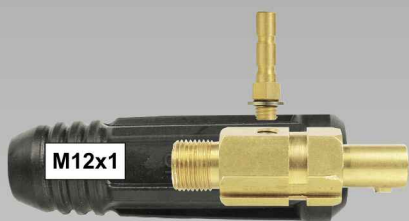
Schweißkabelstecker SK 25 sep. Gasführung
