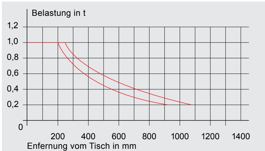
Load diagram, example YHB 1
