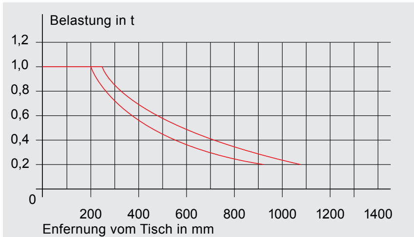
Belastungsdiagramm Beispiel YHB 1
